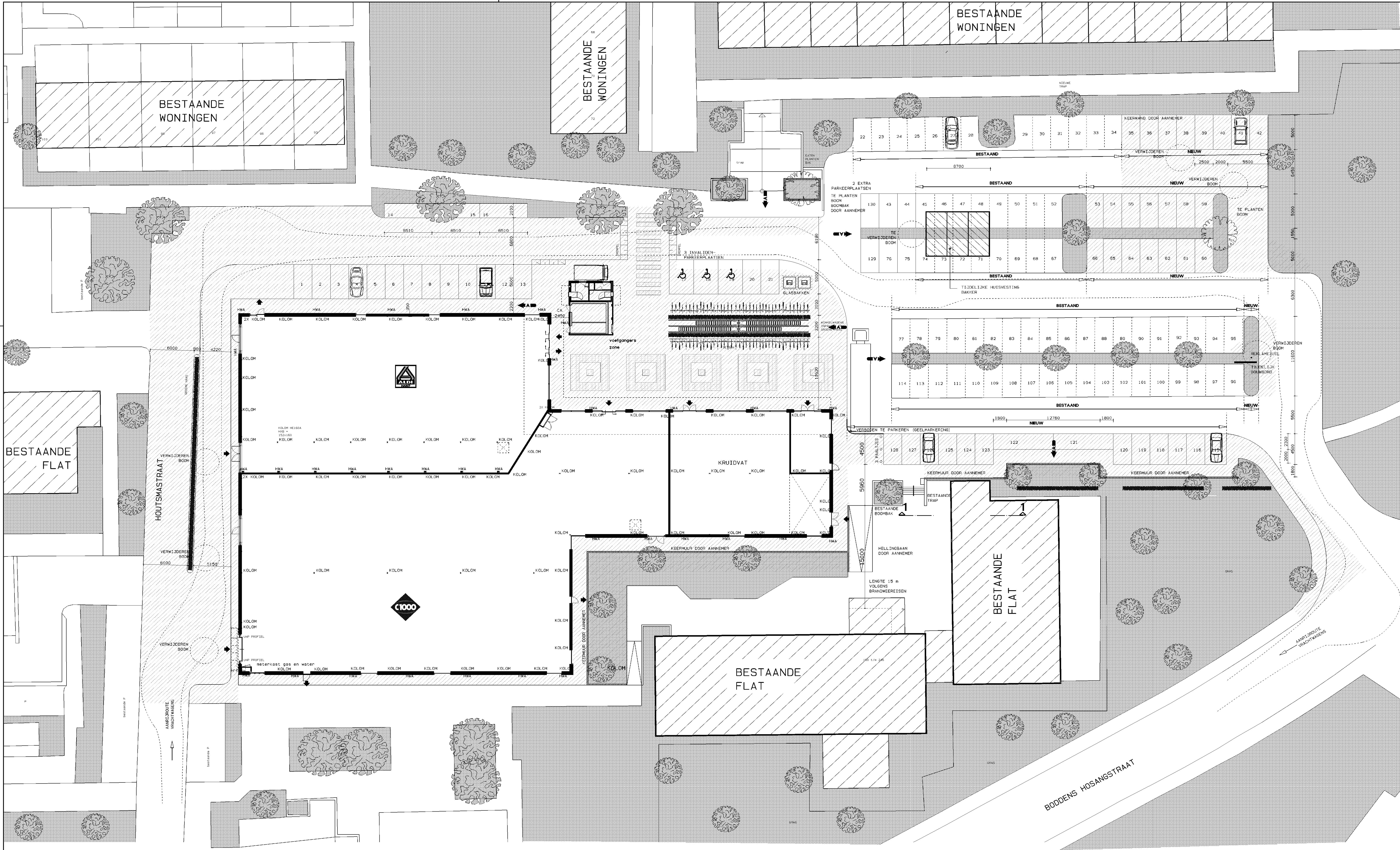
TERREINTEKENING
