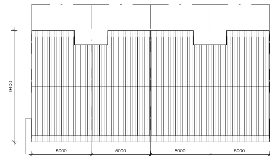
dakverdieping
