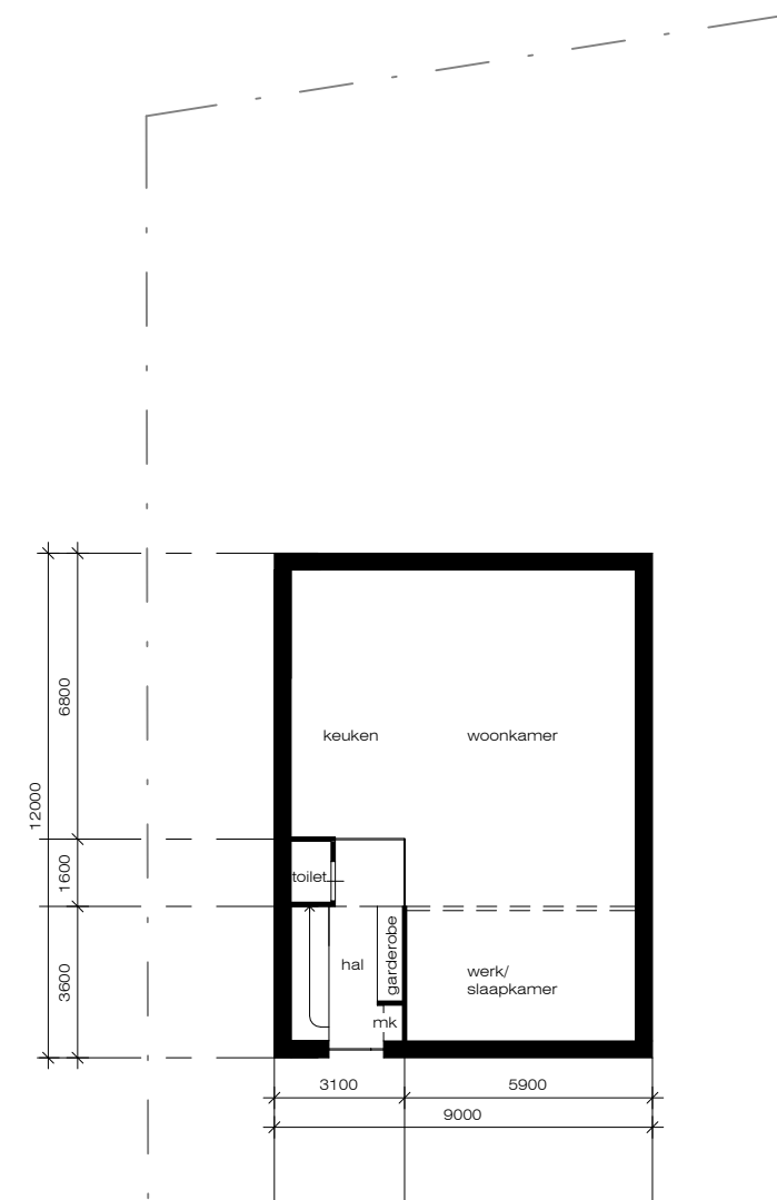
begane grond
